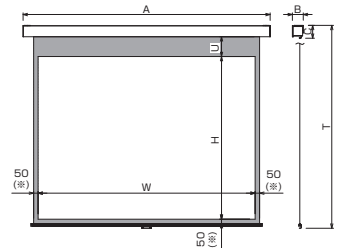
■外形寸法図
