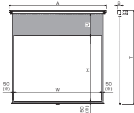
■外形寸法図
