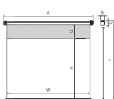
■外形寸法図
