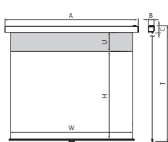
■外形寸法図
