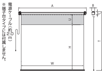
■外形寸法図
