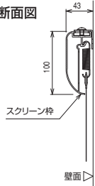
■Z-Z断面図
