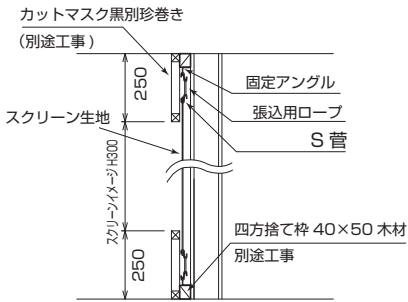
断面詳細図
