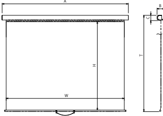
■外形寸法図
