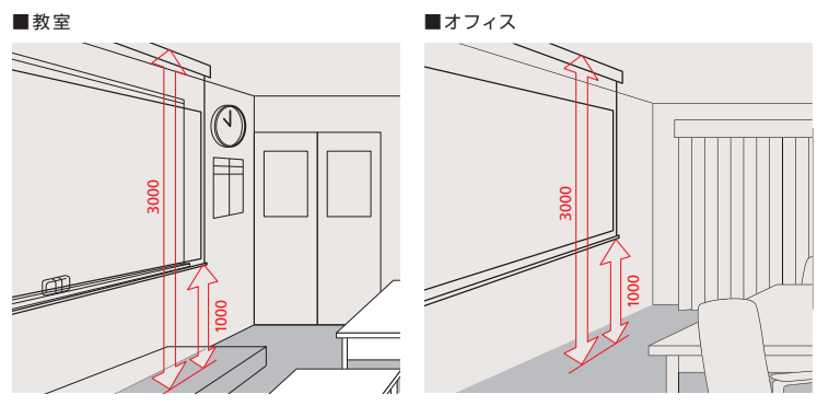
●業務用スクリーン下場は1000を基準とする。(床から黒板の粉受け上面まで)
