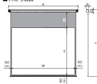
■外形寸法図
