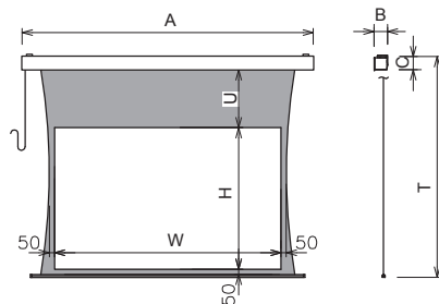
■外形寸法図
