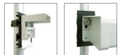
Pセクション スライディングブラケット取付時 Cセクション サイドブラケット取付時
