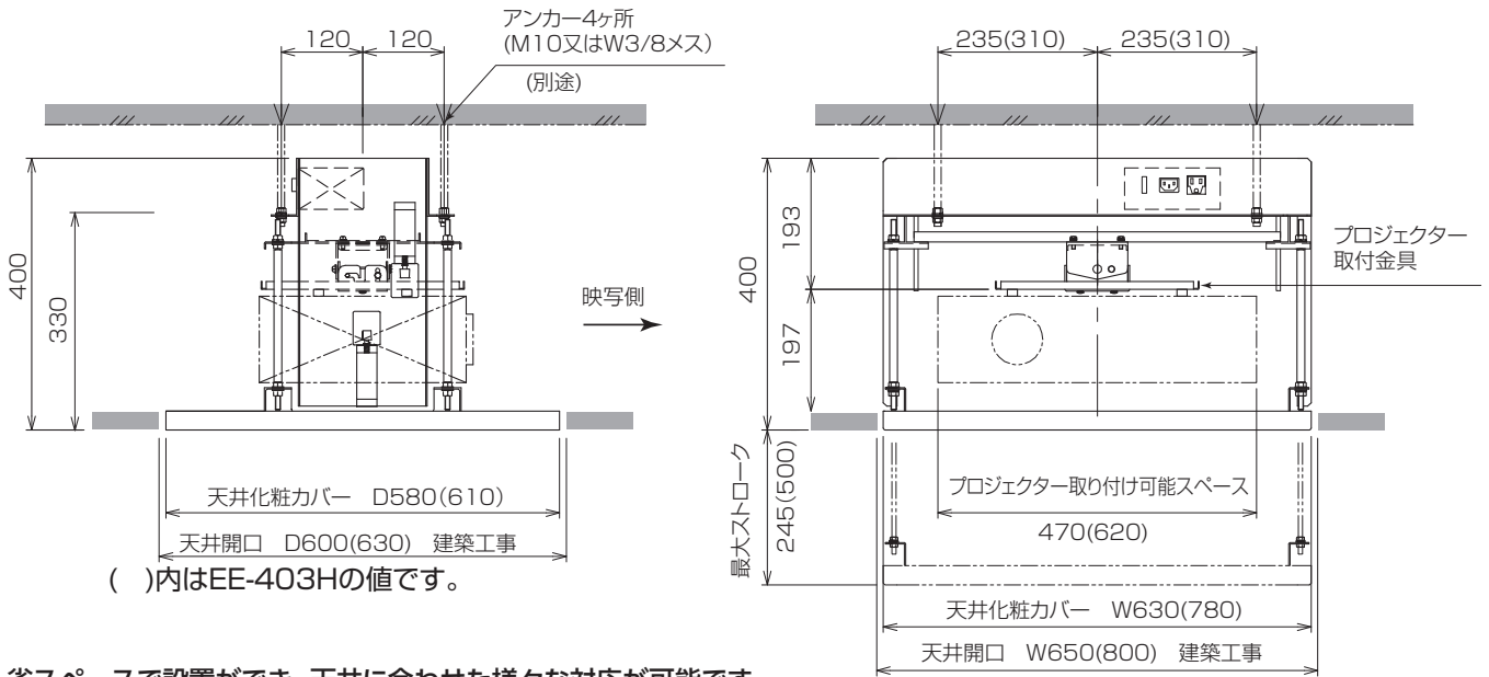
特注:スチールボックス仕上げ、ケーブルガイドはバンタグラフ式
