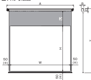
■外形寸法図
