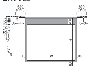
■外形寸法図
