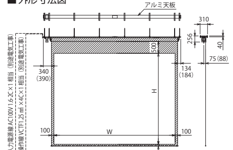
■外形寸法図
