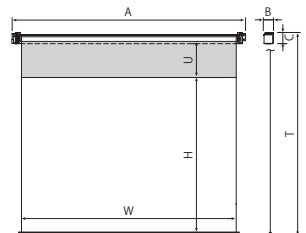
■外形寸法図
