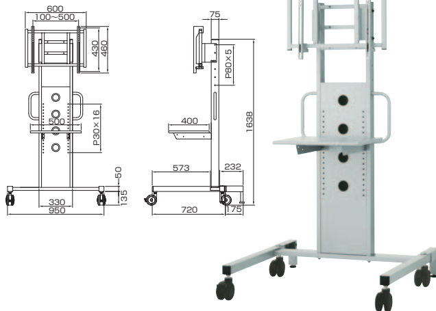
■外形寸法図
