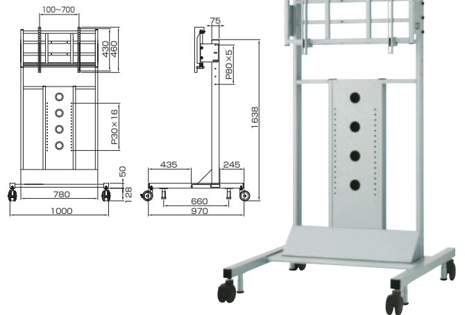
■外形寸法図
