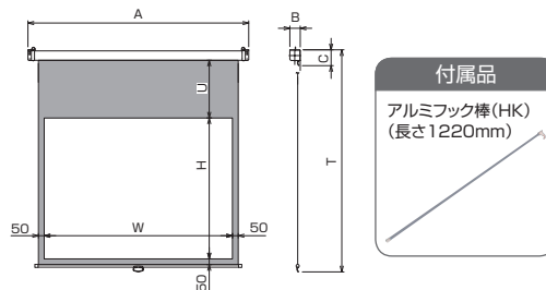
■外形寸法図
