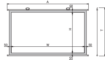
■外形寸法図
