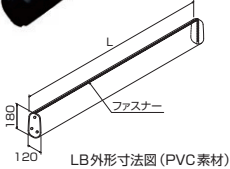
LB外形寸法図 (PVC素材)
