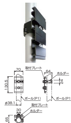
Pセクション スライディングブラケット取付時 Cセクション サイドブラケット取付時
