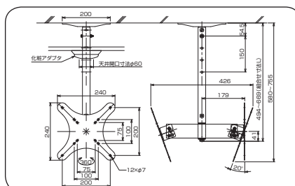
外形寸法図
