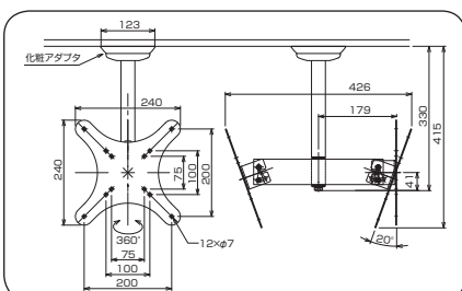
外形寸法図
