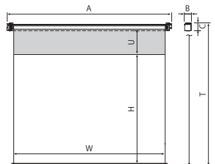
■外形寸法図
