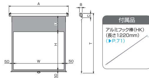
■外形寸法図
