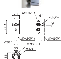
Pセレクション スライディングブラケット取付時
