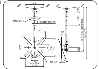
外形寸法図
