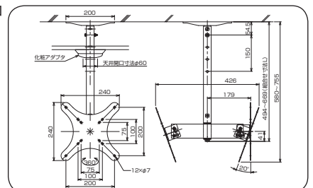
外形寸法図
