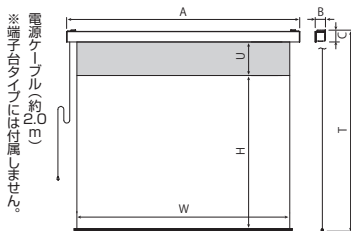
■外形寸法図
