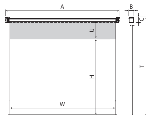
■外形寸法図
