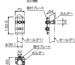
Pセレクション スライディングブラケット取付時
