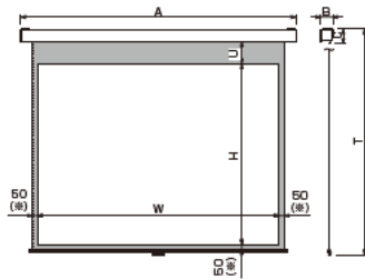
■外形寸法図
