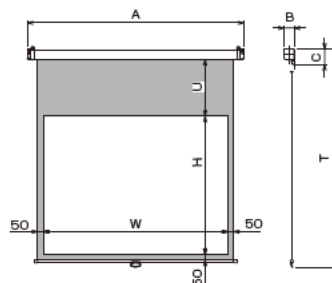
■外形寸法図
