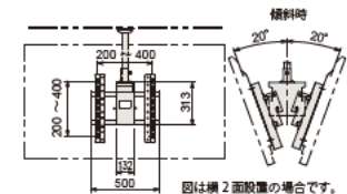
外形寸法図
