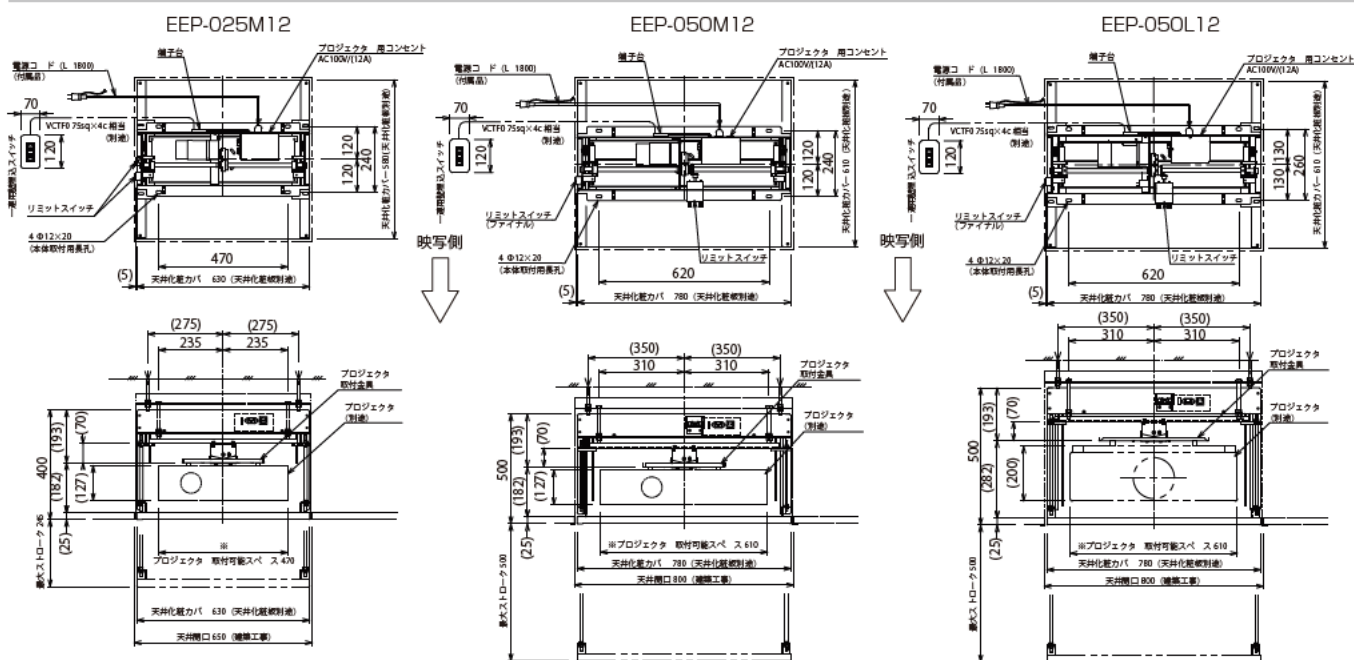
外形寸法図
