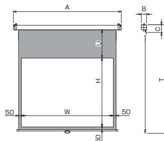
■外形寸法図
