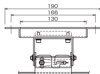
天井取付金具 (前側)
