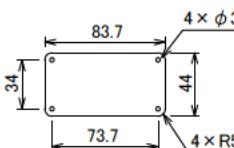
【参考】ブランクパネル(C-FB)寸法図
