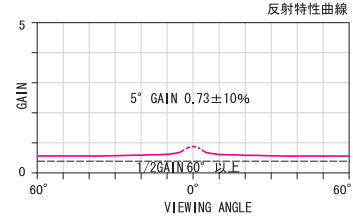
反射特性曲線
