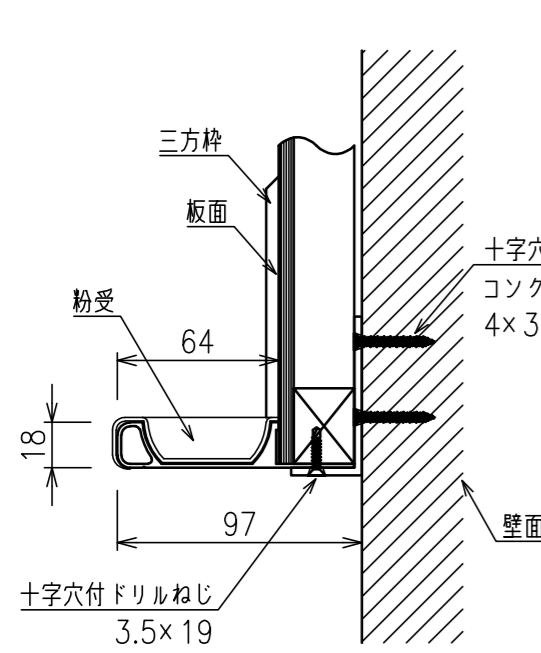
A - A 断面拡大図 S=1:3
