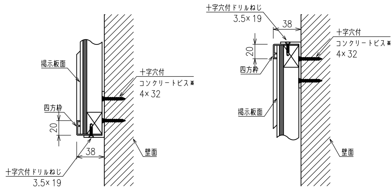
A - A 断面拡大図 S=1:3
