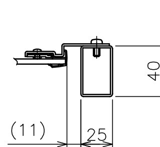
A-A 断面
