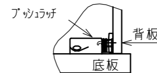
a部詳細
