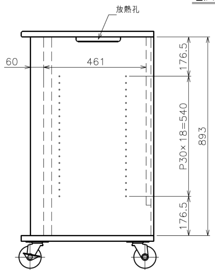
EIA 詳細図
