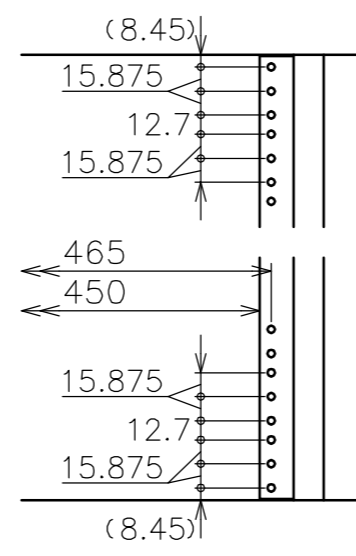
EIA 詳細図
