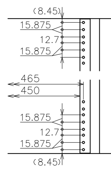
EIA 詳細図
