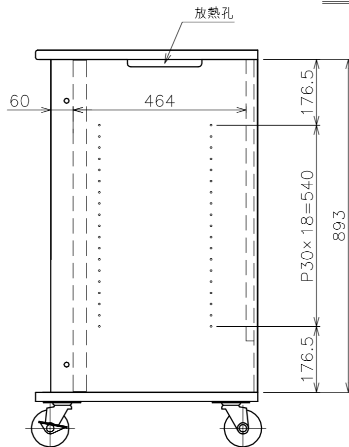
EIA 詳細図
