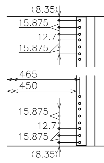
EIA 詳細図
