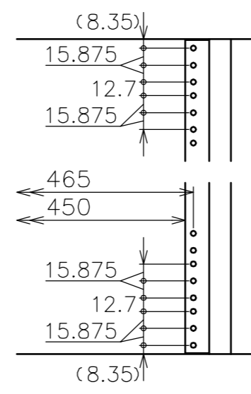
EIA 詳細図
