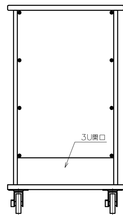
EIA 詳細図
