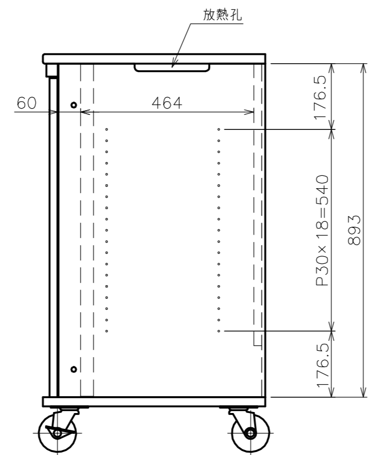
EIA 詳細図
