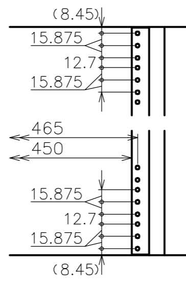
EIA 詳細図
