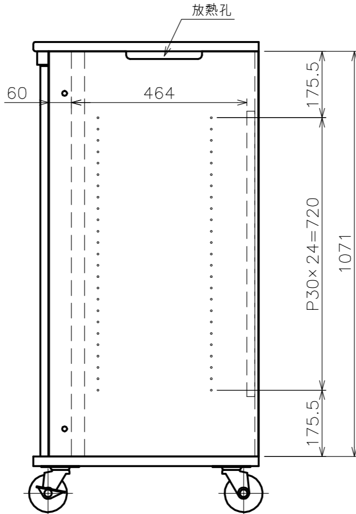
EIA 詳細図
