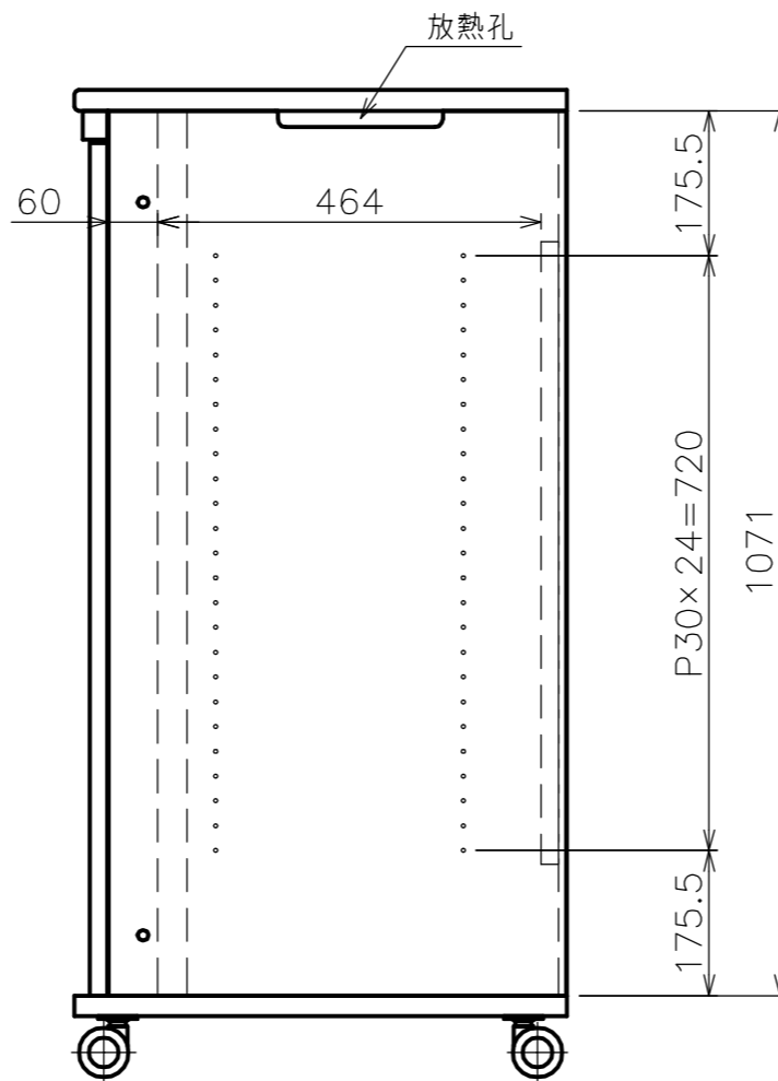
EIA 詳細図
