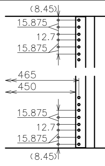
EIA 詳細図
