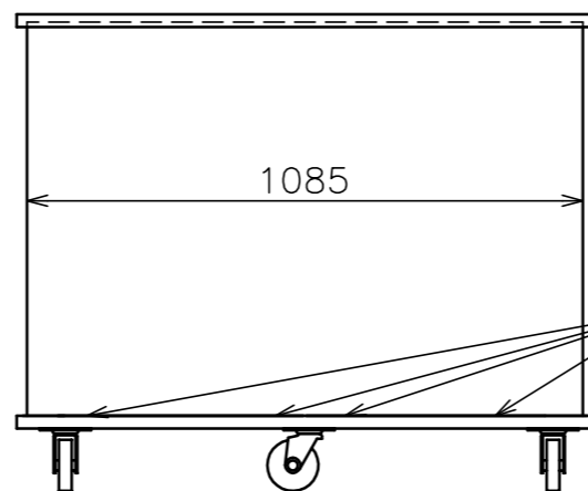
背面図
