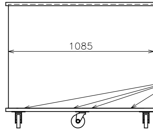
背面図
