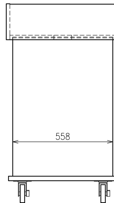
背面図
